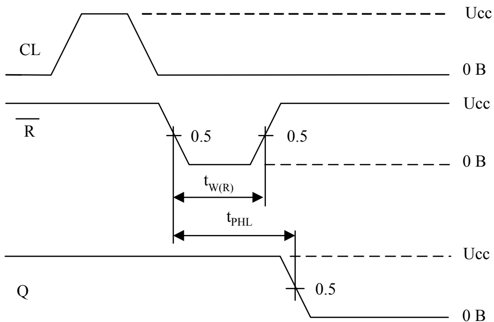
Рисунок 2 – Временная диаграмма входных и выходных импульсов при контроле динамических параметров микросхемы
