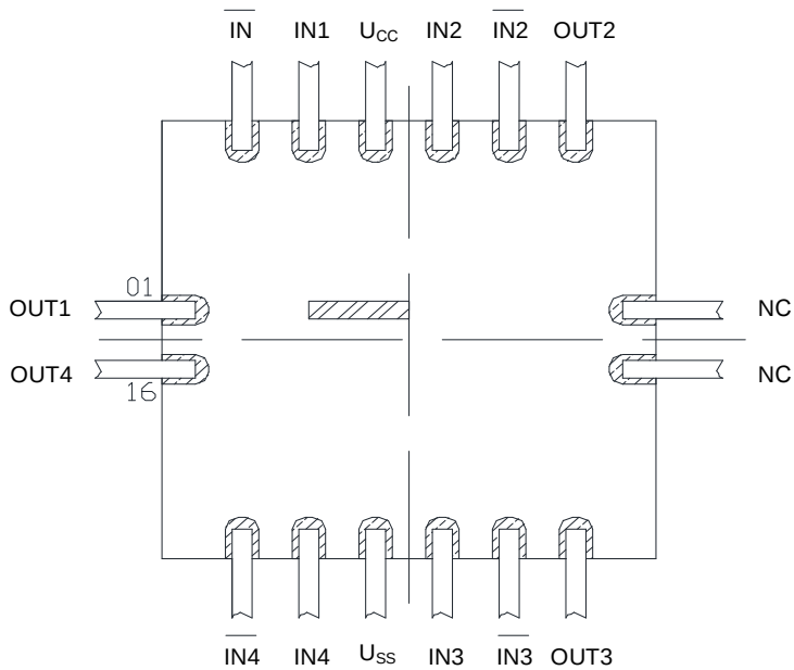
Рисунок 2 – Обозначение выводов в корпусе
