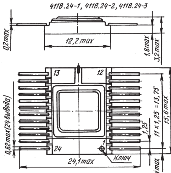
Рисунок 2. Габаритный чертеж корпуса 4118.24-1
