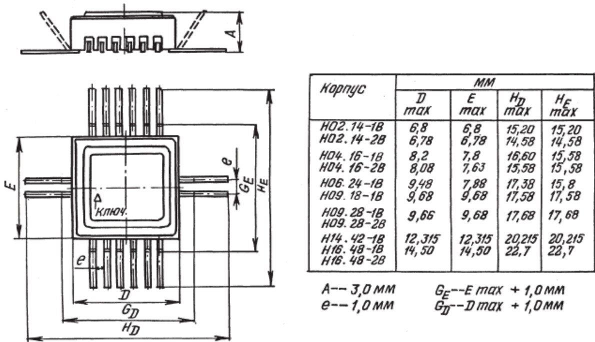
Рисунок 1. Габаритный чертеж корпуса Н14.42-1В
