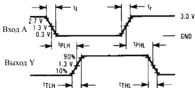
Рисунок 1. Временная диаграмма испытаний
